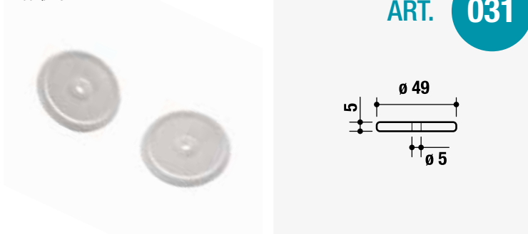
Ruota ø 49 mm Wheel ø 49 mm
